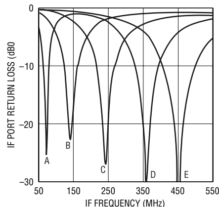
5557 G09 A: 70MHz, L1 = 270nH, C3 = 15pF B: 140MHz, L1 = 180nH, C3 = 3.9pF C: 240MHz, L1 = 82nH, C3 = 2.2pF D: 360MHz, L1 = 47nH, C3 = 1.2pF E: 450MHz, L1 = 39nH, C3 = 0pF
